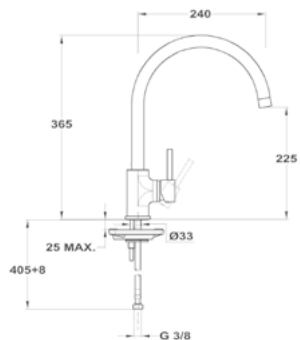
Evo X mosogató csapterep 152-0052-01
